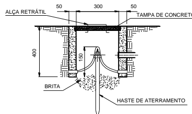
CORTE AA'
